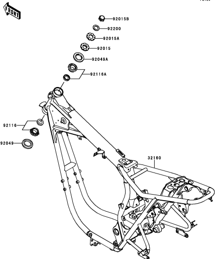
E-3 Frame 1 1 2 2 3 3 4 4 5 5 6 6 7 7 8 8 9 9 10 10 11 11 12 12 13 13 14 14 15 15 16 16 17 17 18 18 19 19 20 20 21 21 22 22 23 23 24 24 25 25 26 26 27 27 28 28 29 29 30 30 31 31 32 32 33 33 34 34 35 35 36 36 37 37 38 38 39 39 40 40 41 41 42 42 43 43 44 44 45 45 46 46 47 47 48 48 49 49 50 50 51 51 52 52 53 53 54 54 55 55 56 56 57 57 58 58 59 59 60 60 61 61 62 62 63 63 64 64 65 65 66 66 67 67 68 68 69 69 70 70 71 71 72 72 73 73 74 74 75 75 76 76 77 77 78 78 79 79 80 80 81 81 82 82 83 83 84 84 85 85 86 86 87 87 88 88 89 89 90 90 91 91 92 92 93 93 94 94 95 95 96 96 97 97 98 98 99 99 100 100
