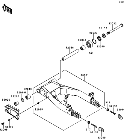
E-3 Frame 1 1 2 2 3 3 4 4 5 5 6 6 7 7 8 8 9 9 10 10 11 11 12 12 13 13 14 14 15 15 16 16 17 17 18 18 19 19 20 20 21 21 22 22 23 23 24 24 25 25 26 26 27 27 28 28 29 29 30 30 31 31 32 32 33 33 34 34 35 35 36 36 37 37 38 38 39 39 40 40 41 41 42 42 43 43 44 44 45 45 46 46 47 47 48 48 49 49 50 50 51 51 52 52 53 53 54 54 55 55 56 56 57 57 58 58 59 59 60 60 61 61 62 62 63 63 64 64 65 65 66 66 67 67 68 68 69 69 70 70 71 71 72 72 73 73 74 74 75 75 76 76 77 77 78 78 79 79 80 80 81 81 82 82 83 83 84 84 85 85 86 86 87 87 88 88 89 89 90 90 91 91 92 92 93 93 94 94 95 95 96 96 97 97 98 98 99 99 100 100
