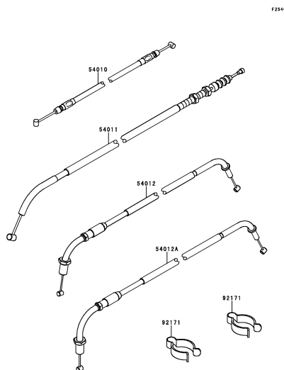
F-10 Cables
